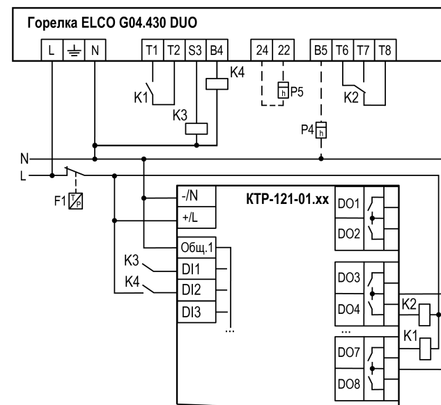
Рисунок В.4 – Пример подключения двухступенчатой горелки ELCO G04.430 DUO к KTR-121.01.10
