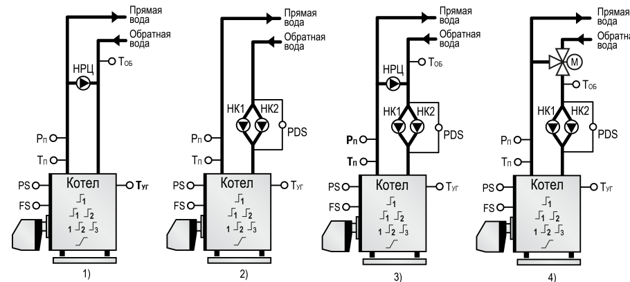
Рисунок 1.1 – Объект управления
