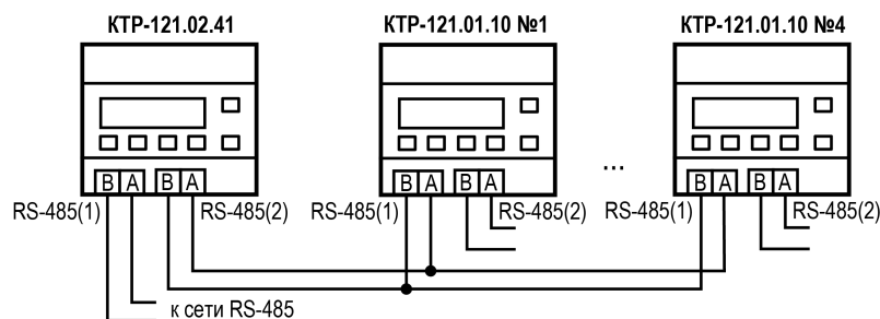
Рисунок 5.1 – Соединение ведущего КТР-121 и подчиненных приборов
